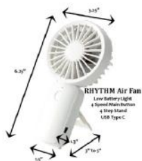
Dimensions
